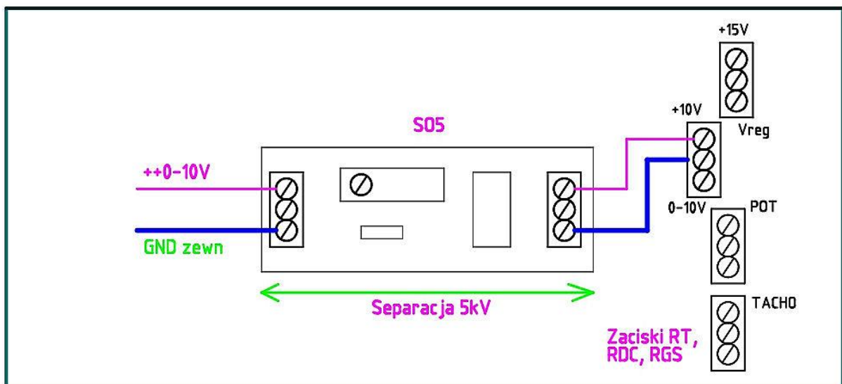
Schemat podłączenia separacji optycznej
